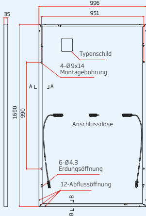
Rückansicht (Hochformat)
